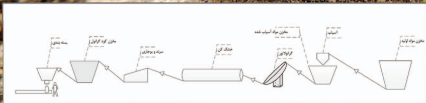
خط تولید کود گرانول
