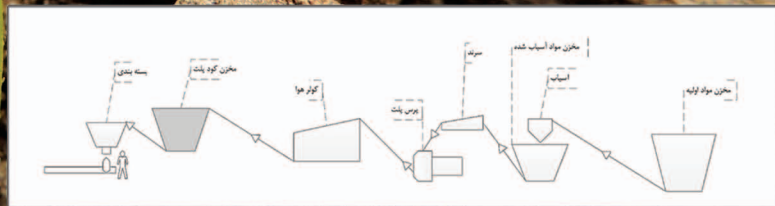
خط تولید کود پلت
